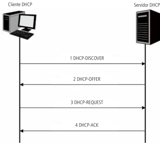
Negociação DHCP
