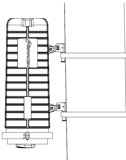
FIXAÇÃO EM POSTE ATRAVÉS DE FITA DE AÇO INOXIDÁVEL
